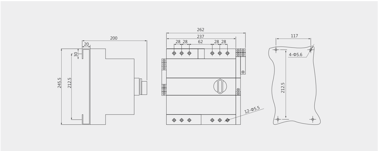
KB1S-125 四极双电源自动转换开关
