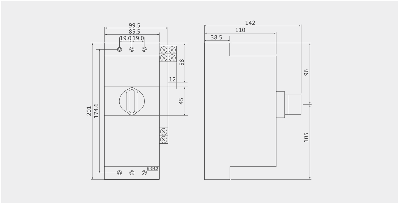
四极 KB1-45 型安装尺寸
