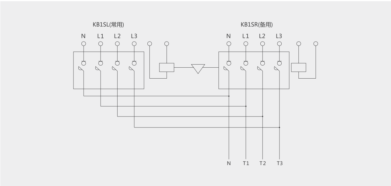
KB1S 双电源自动转换开关 PC 级电气原理图（图二）
