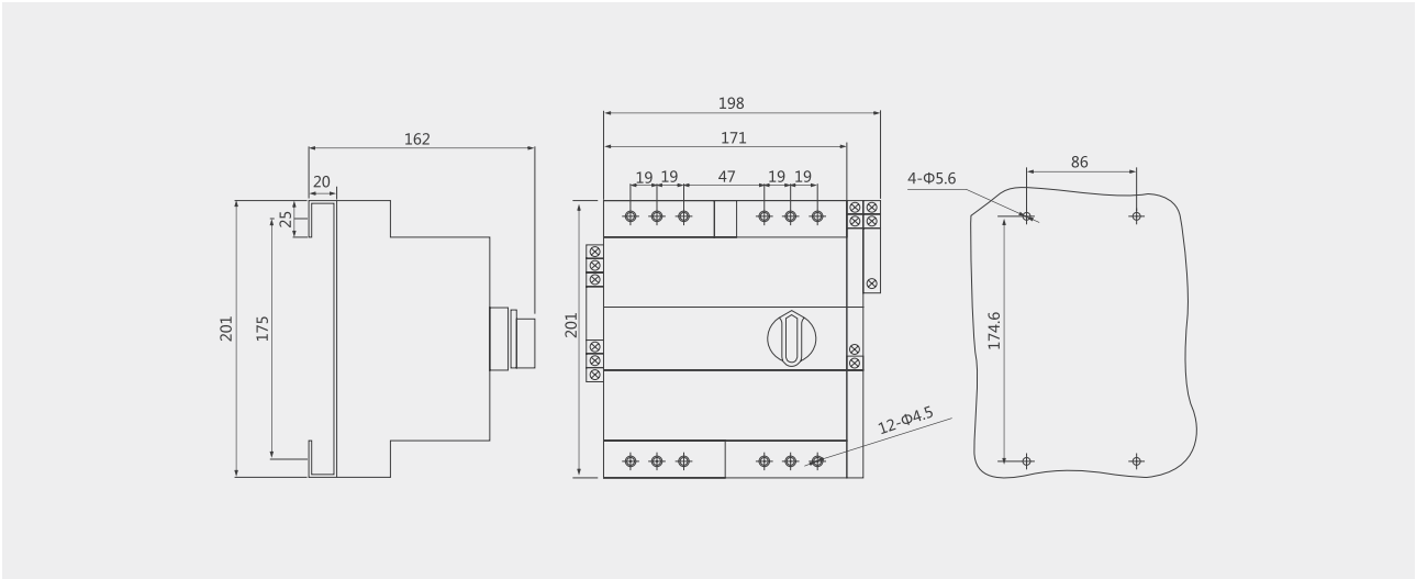
KB1S-45 四极双电源自动转换开关
