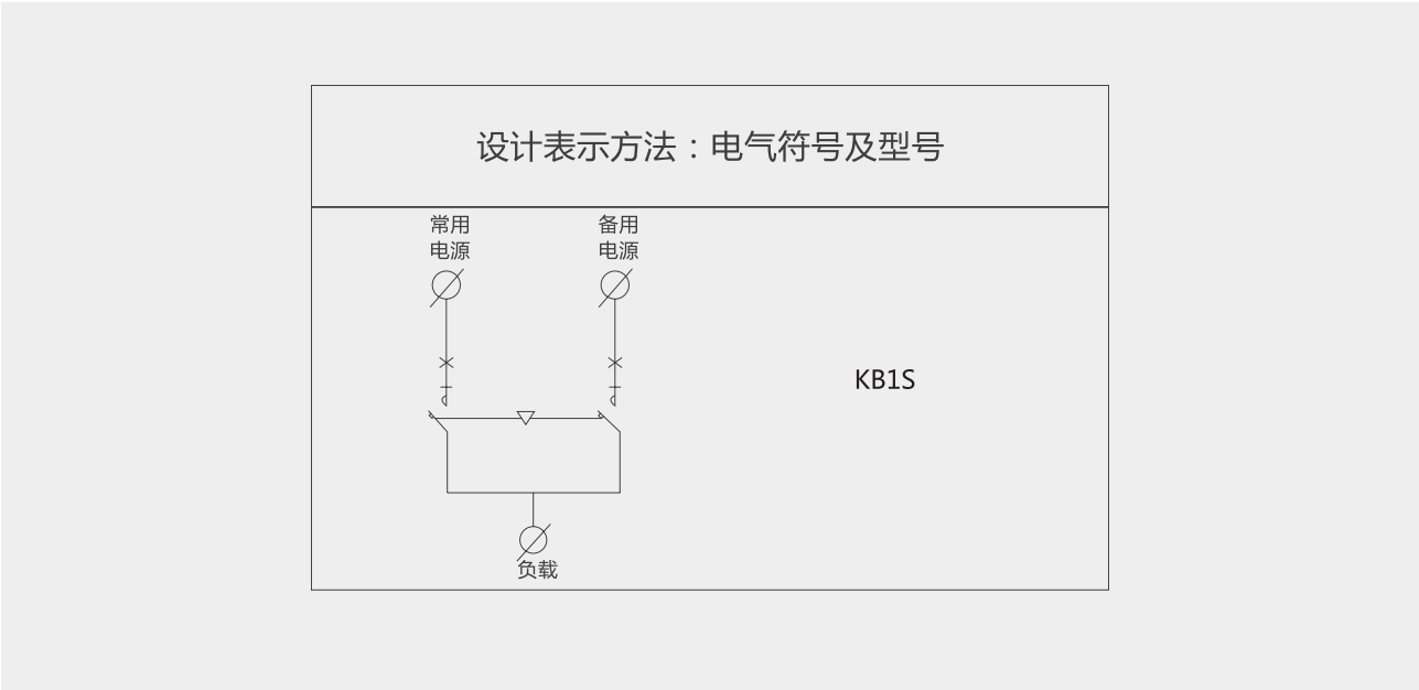
电气设计表示方法（图一）
