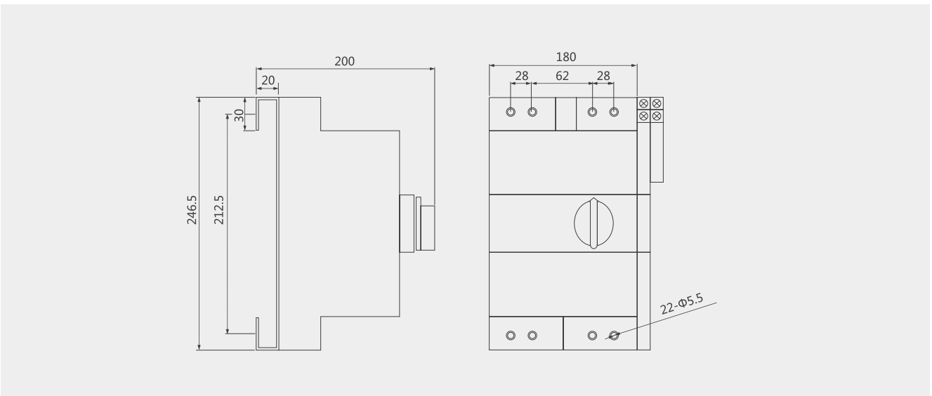
KB1S-125 三极双电源自动转换开关
