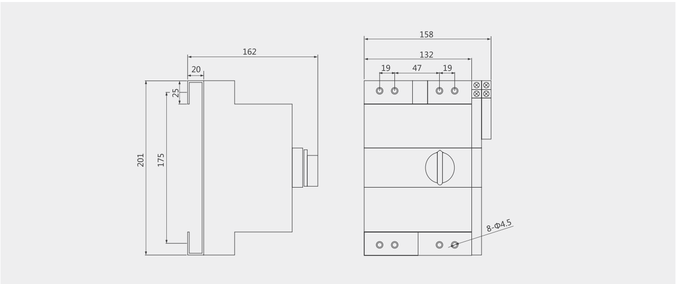
KB1S-45 三极双电源自动转换开关
