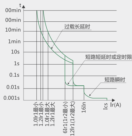
电动机保护曲线图
