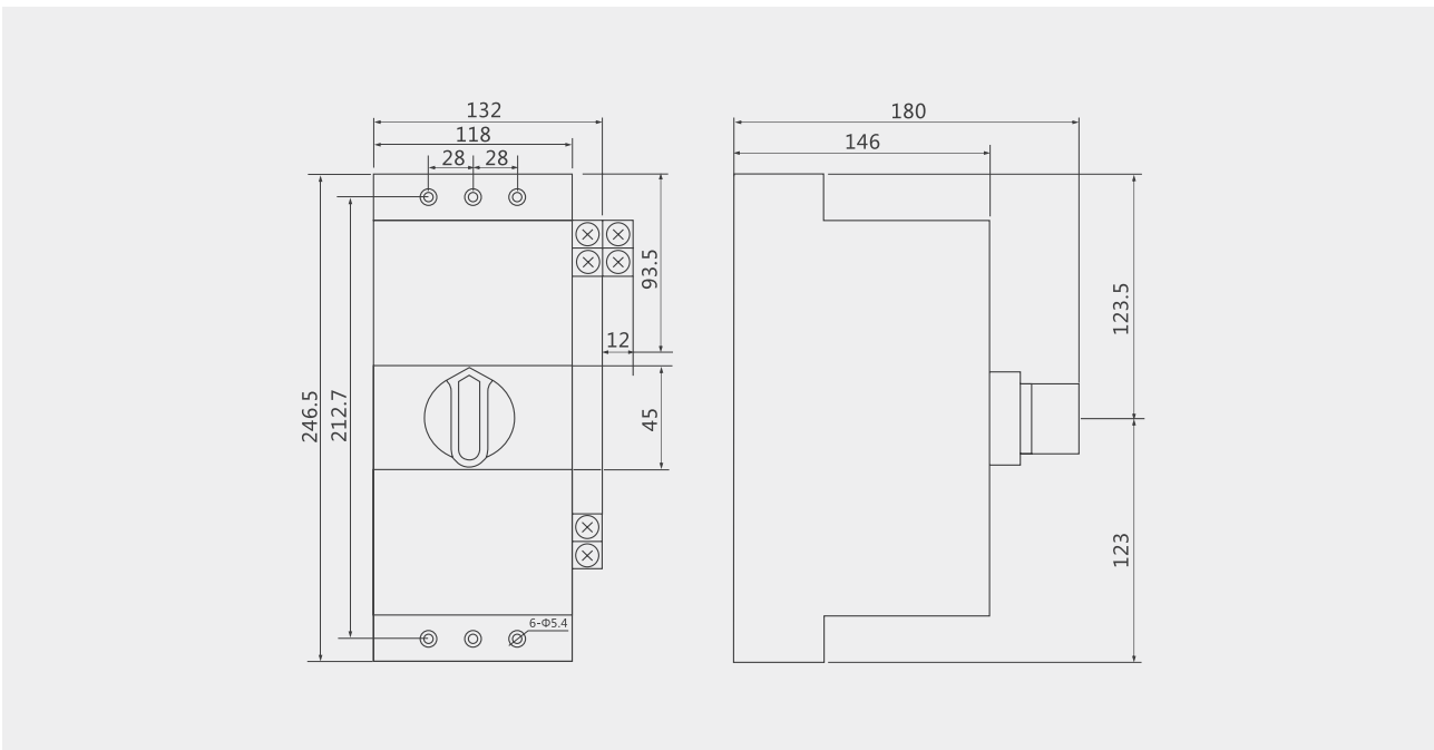
四极 KB1-125 型安装尺寸
