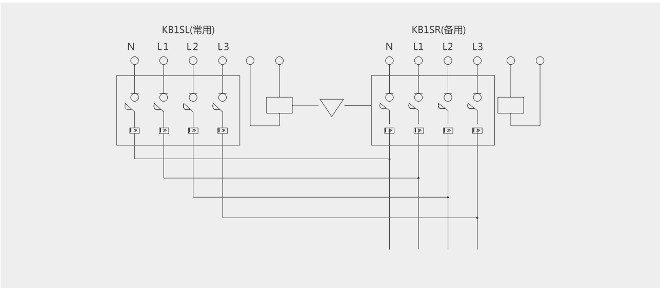
KB1S 双电源自动转换开关 CB 级电气原理图（图三）
