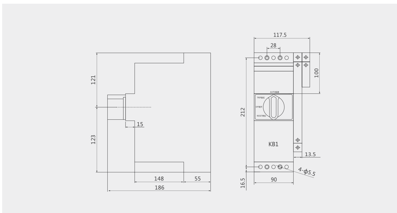
KB1-125 型安装尺寸
