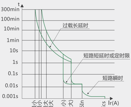
配电保护曲线图
