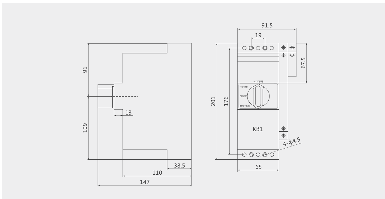
KB1-45 型安装尺寸
